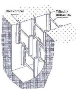
Apuntalamiento Hidráulico Vertical de Aluminio (Apilado)
