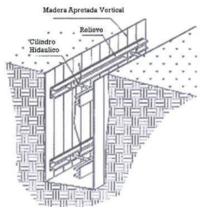
Sistema de agua de apuntalamiento hidráulico de aluminio (Típico)
