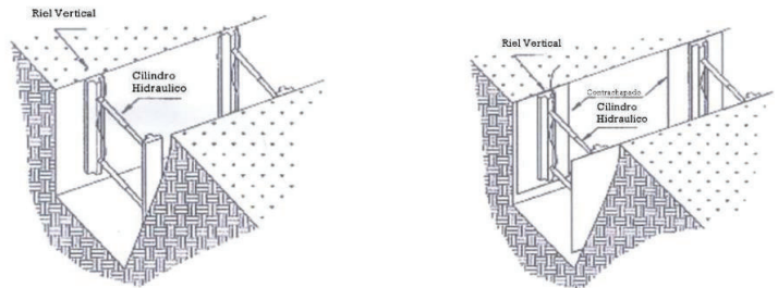
Apuntalamiento Hidráulico Vertical de Aluminio (Refuerzos puntuales)
